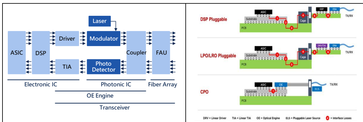
圖 10：光收發模組(左)；插拔式光收發模組、LPO 架構、CPO 架構均需外接插拔式光模組(右)
